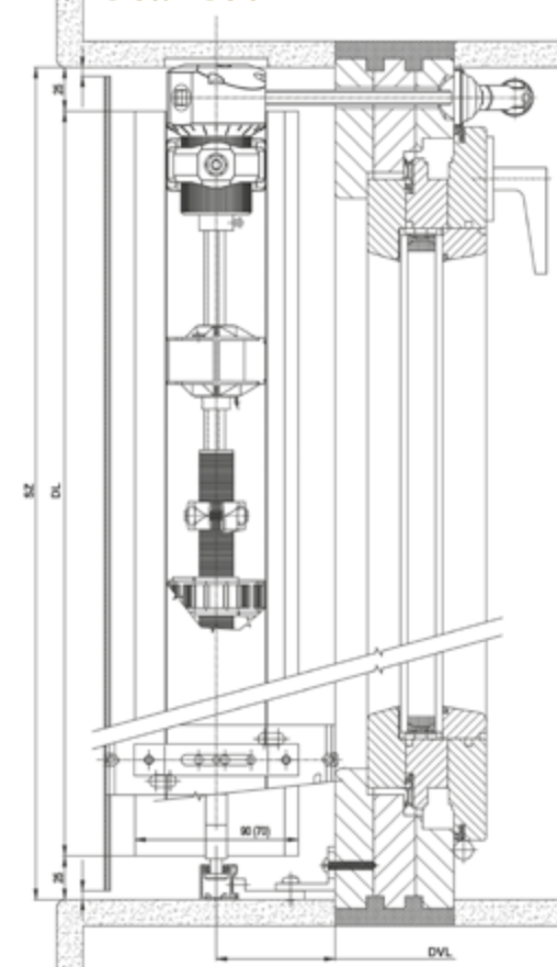
Détail BSO
